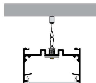
Κρέμαστη τοποθέτηση με σκέτ κρέμανσης Pendant installation with hanging Kit
