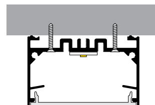
Επίτοιχη τοποθέτηση Surface mounted installation
