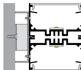
Διπλή τοποθέτηση με ροζέτα Double installation with rosette
